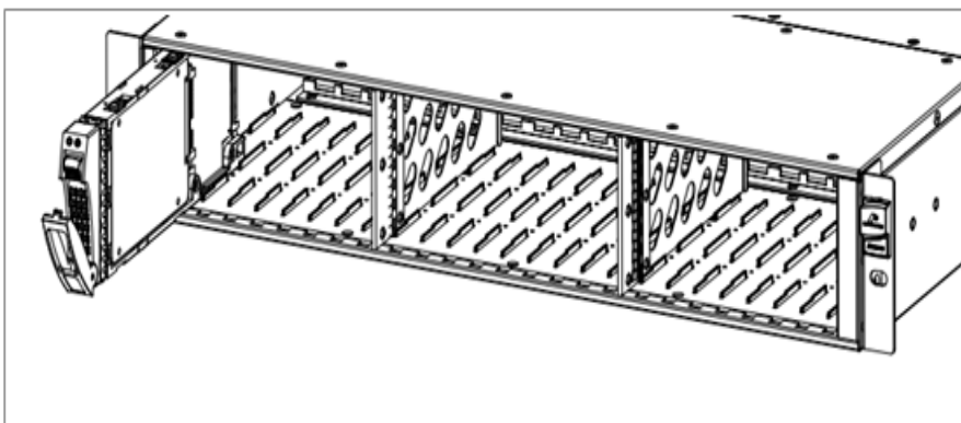
图6-15 安装 2.5 英寸磁盘模块示意图（二）
