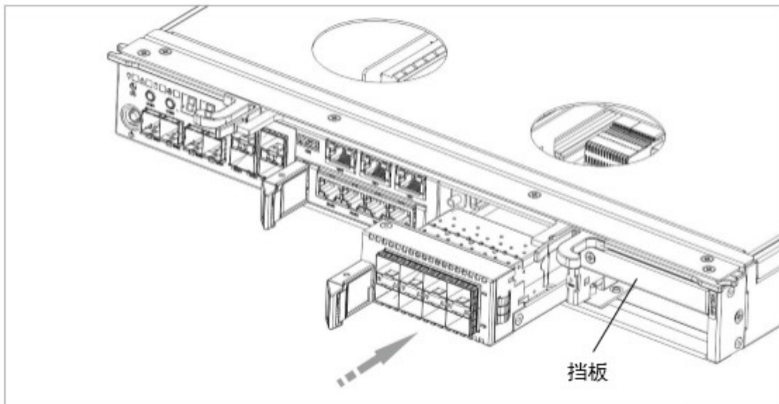
图6-10 安装/拆卸 IO 插卡大卡示意图
