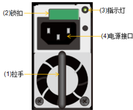
图3-16 DSU2624 电源模块正视图
