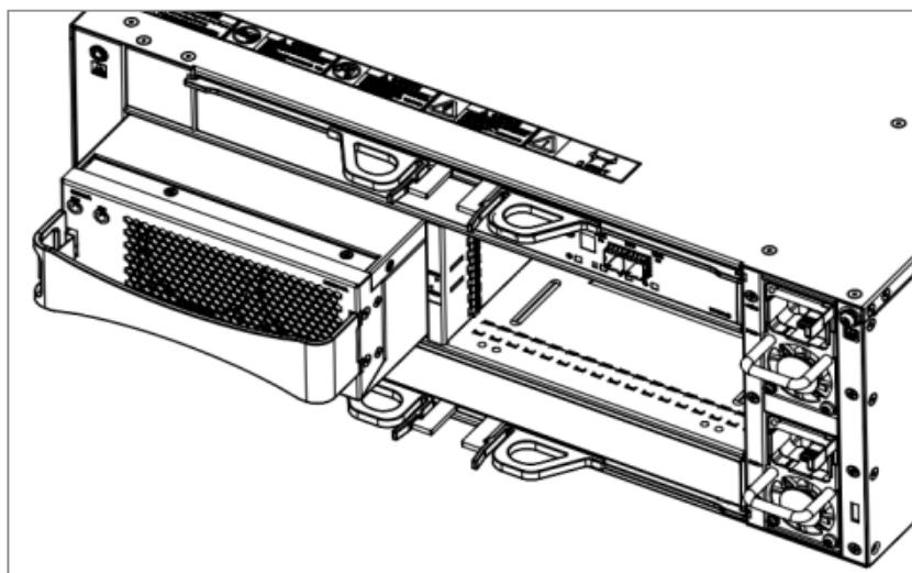
图6-8 安装/拆卸 DSU2624 风扇模块示意图
