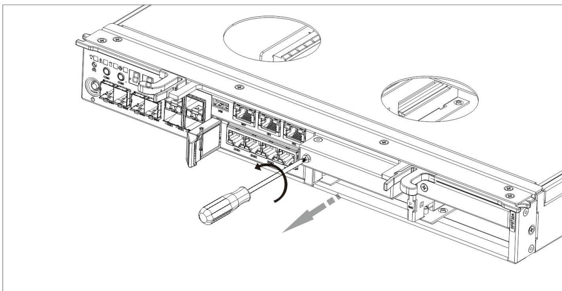
图6-11 拆卸挡板示意图
