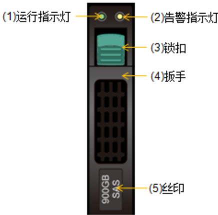
图3-17 2.5 英寸磁盘模块前面板
