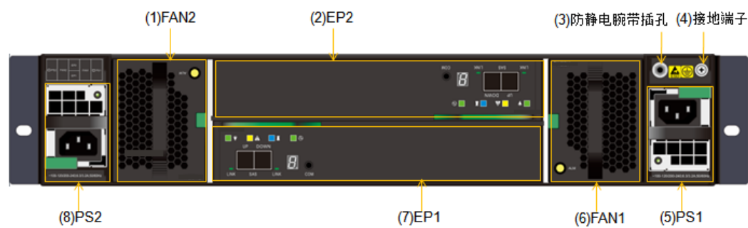
图3-8 DSU2625 后正视图
